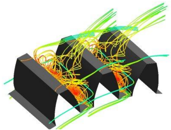
Ecoulement au passage d'une roue dentée - pertes aérodynamiques dans les transmissions mécaniques
